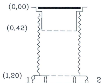
Šulinio pjūviai
