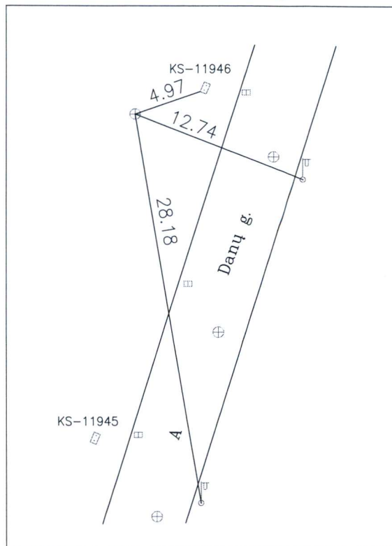
Pririšimo brėžinys
