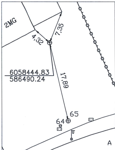
PRIRIŠIMO BRĖŽINYS
