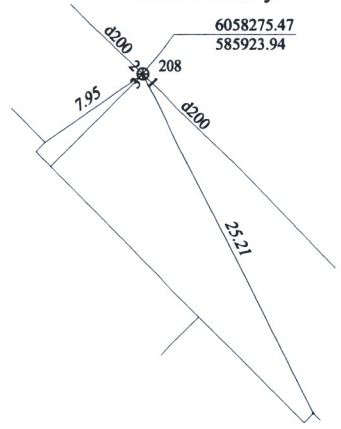
Pririšimo brėžinys
