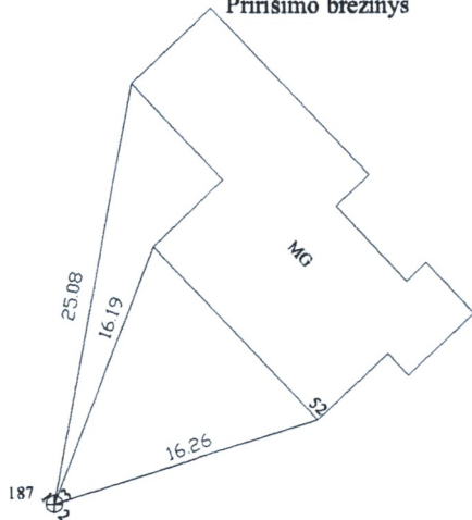
Prišimo brėžinys
