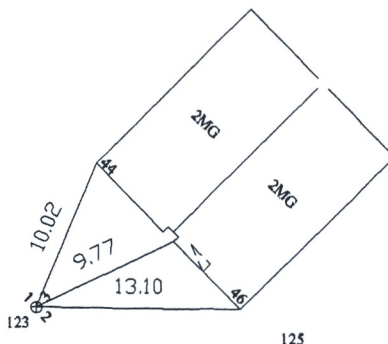
Pririšimo brėžinys
