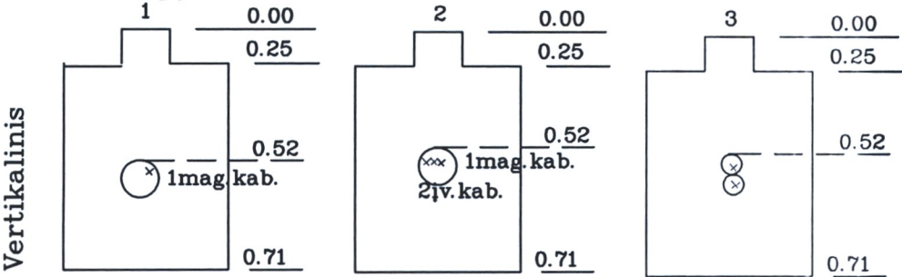
Šulinio pjūviai :
