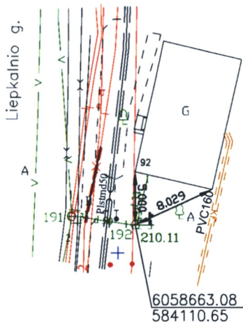
Pririšimo brėžinys
