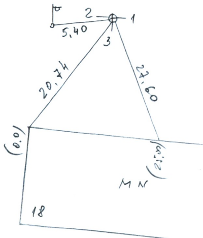
PRIRIŠIMO SCHEMA
