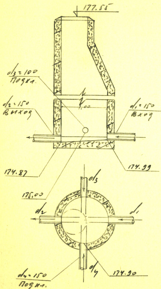
Чертеж колодца М 1:50
