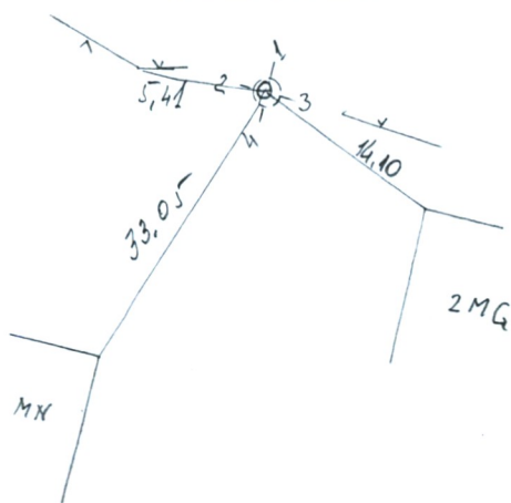
PRIRIŠIMO SCHEMA
