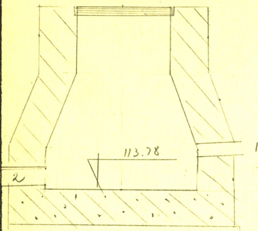
Чертеж колодца М 1:
