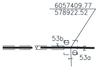
Pririšimo brėžinys
