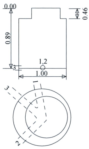
Šulinio pjūviai
