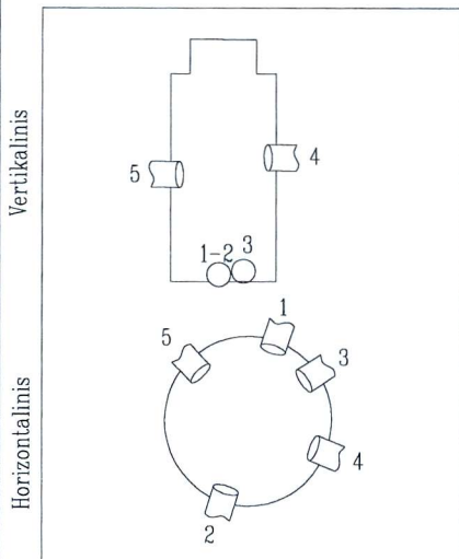
ŠULINIO PĖJŲIAI (Matmenys duoti m)
