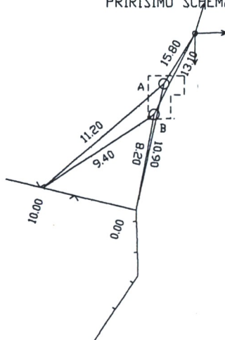
PRIRIŠIMO SCHEMA
