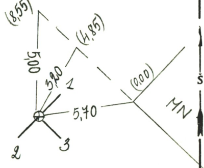
PRIRIŠIMO BRĖŽINYS
