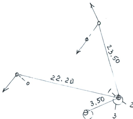
PRIRIŠIMO SCHEMA
