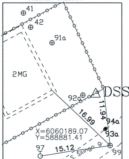
PRIRIŠIMO BRĖŽINYS
