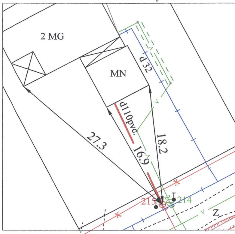
Pririšimo brėžinys
