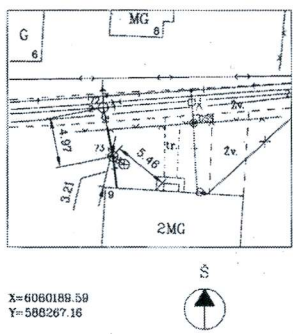
Pririšimo brėžinys :
