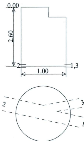
Šulinio pjūviai
