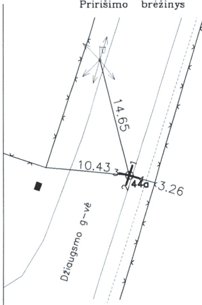
Pririšimo brėžinys
