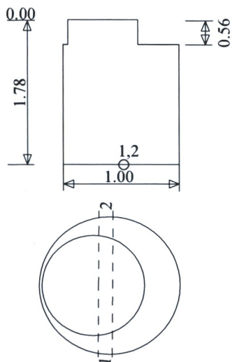
Šulinio pjūviai
