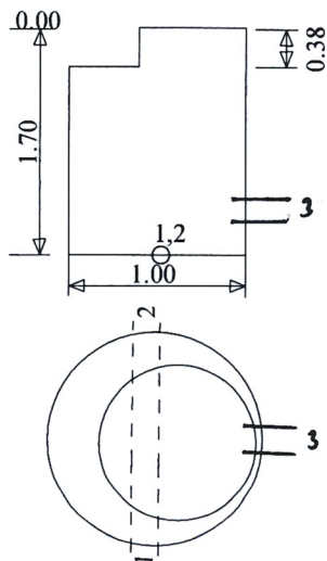
Šulinio pjūviai
