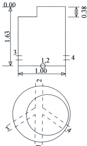
Šulinio pjūviai
