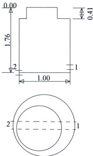
Šulinio pjūviai
