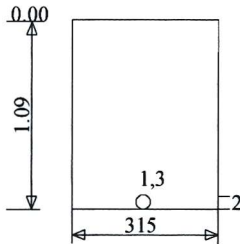
Šulinio pjūviai
