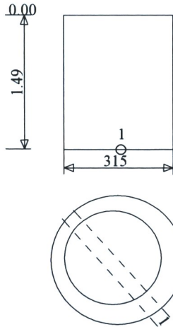
Šulinio pjūviai
