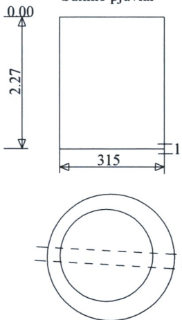
Šulinio pjūviai
