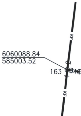
Pririšimo brėžinys
