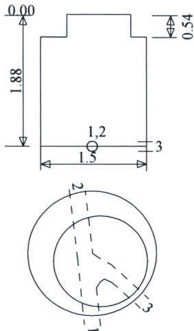
Šulinio pjūviai
