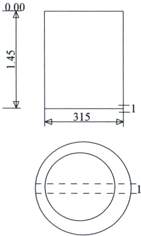
Šulinio pjūviai
