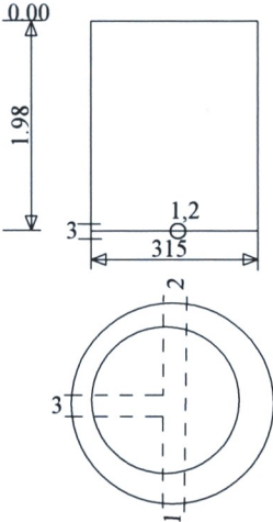
Šulinio pjūviai
