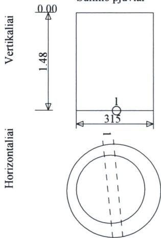
Šulinio pjūviai
