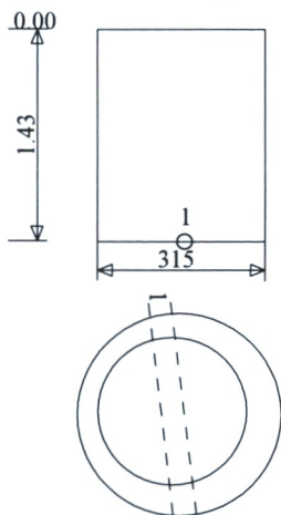
Šulinio pjūviai
