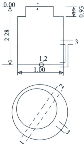
Šulinio pjūviai
