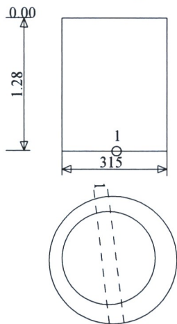
Šulinio pjūviai
