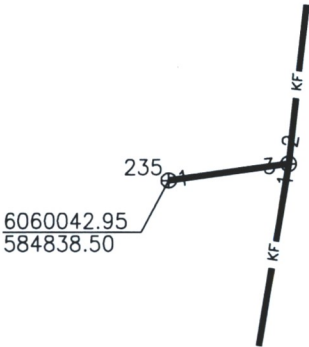
Pririšimo brėžinys
