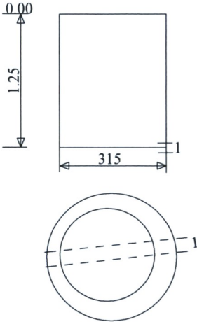
Šulinio pjūviai
