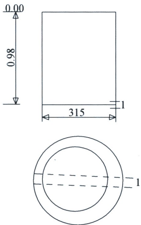
Šulinio pjūviai
