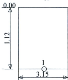
Šulinio pjūviai
