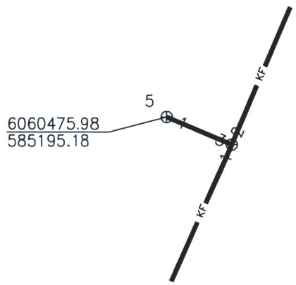
Pririšimo brėžinys
