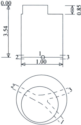
Šulinio pjūviai
