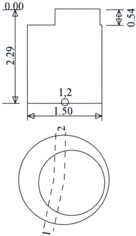
Šulinio pjūviai
