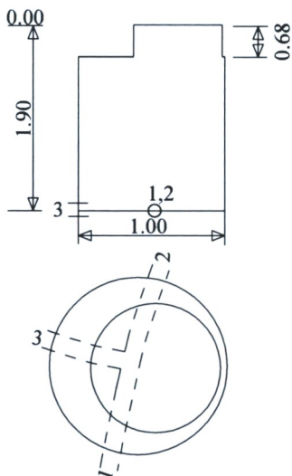
Šulinio pjūviai
