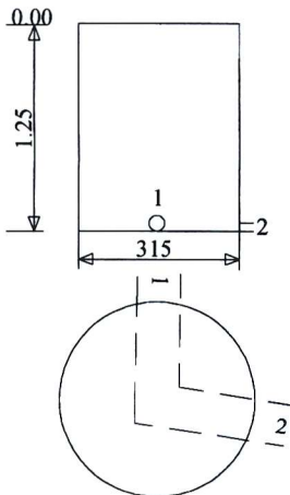
Šulinio pjūviai
