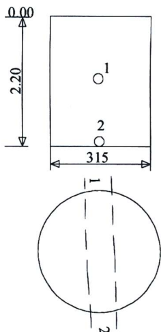
Šulinio pjūviai
