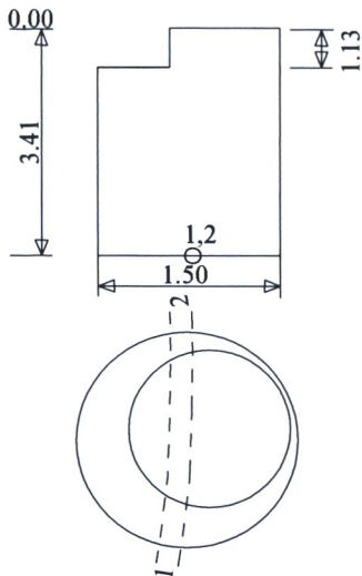
Šulinio pjūviai
