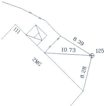
Pririšimo schema
