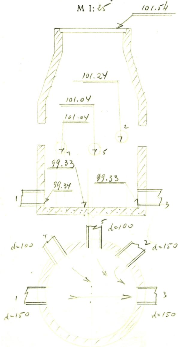
Šulinio brėžinys
