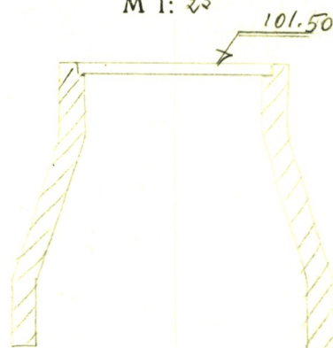
Šulinio brėžinys
